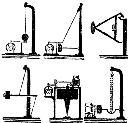
Сейсмографы разных систем
